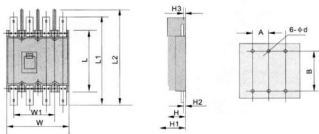
DZ20四极断路器(板前接线)
