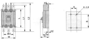
DZ20Y.J.G.C(板后接线)
