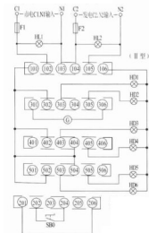
CHCH40-125-630A带发电机接线
