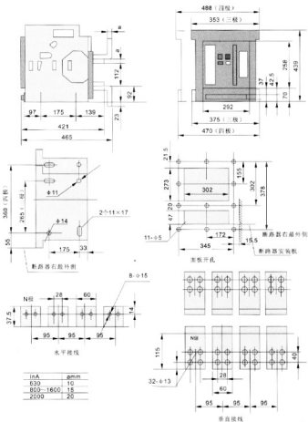
图7-1HCW1-2000 抽屉式
