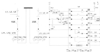
图6-6单路受电操作回路
