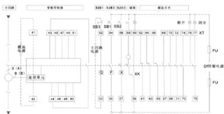
图6-3 1000A壳架断路器接线图 二次回路接线图
